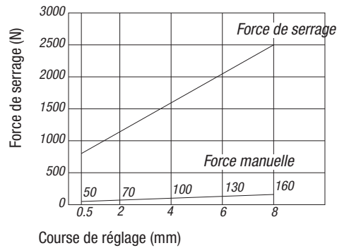
Vérin à tirer K0910.4050...
