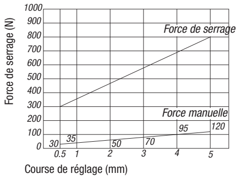
Bride pivotante K0912....3232
