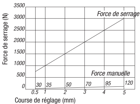
Crampon plaqueur K0928.0500 Crampon plaqueur K0928.0501
