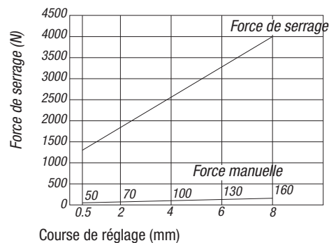
Crampon plaqueur K0928.0800 Crampon plaqueur K0928.0801
