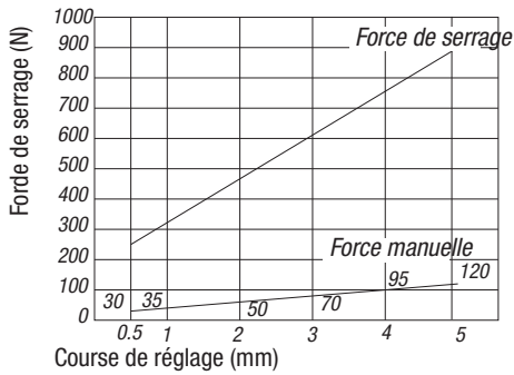
Vérin à tirer K0910.3240...
