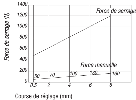
Bride pivotante K0912....4540
